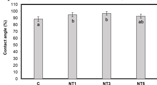
FIGURE 2 Contact angle of samples: (C) Control, (NT1) 1%Nano TiO 2 , (NT3) 3%Nano TiO 2 , (NT5) 5%Nano TiO 2 .
