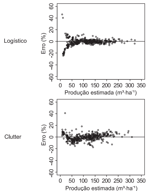
FIGURA 3 Distribuição dos resíduos, em porcentagem, em função do volume estimado de madeira para celulose para o modelo Logístico e modelo de Clutter.
