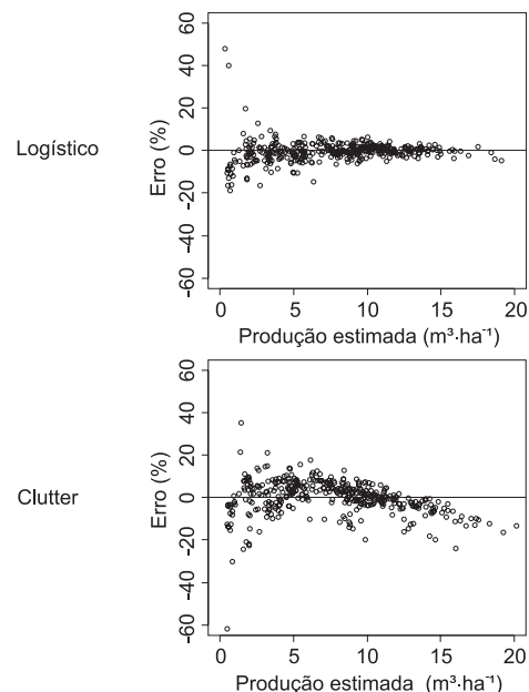
FIGURA 2 Distribuição dos resíduos, em porcentagem, em função do volume estimado de madeira para energia para o modelo Logístico e modelo de Clutter.
