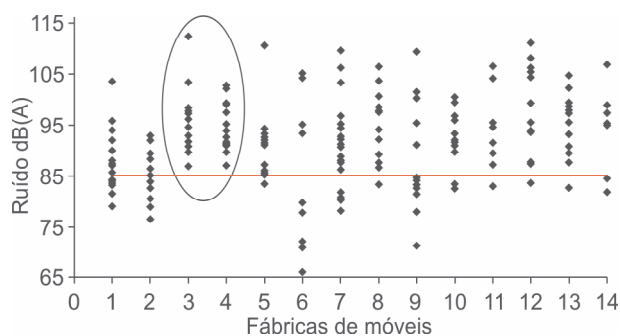
FIGURA 2 Disposição dos valores de ruído em relação ao limite estabelecido pela NR- 15, para 8 horas de trabalho (BRASIL, 2008).
